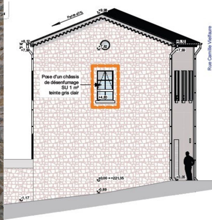
Façade Nord-Est_PRO_Rue des Pénitents
